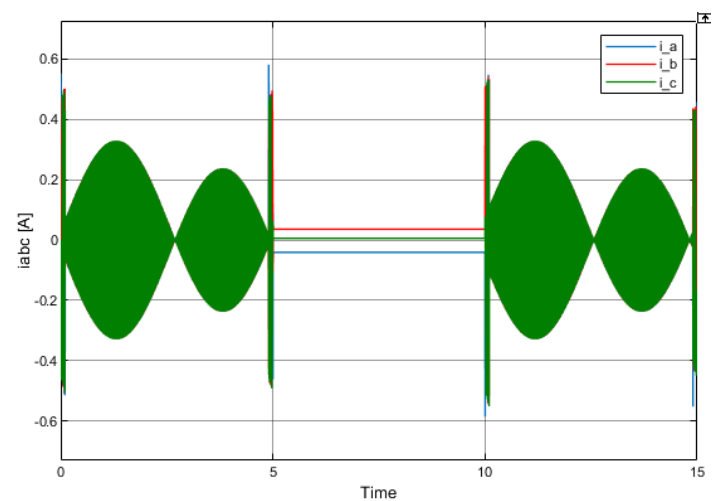
Figura 56: Corrientes i_{abc}
