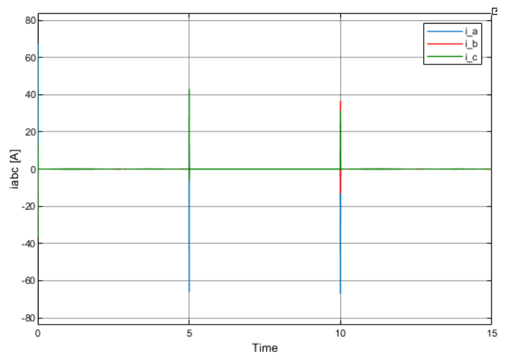
Figura 46: Corrientes i_{abc}(t)
