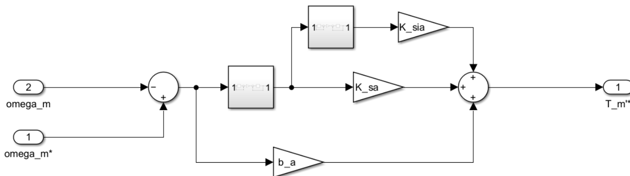
Figura 91: PID externo discretizado
